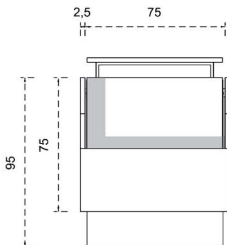
PIANTA
