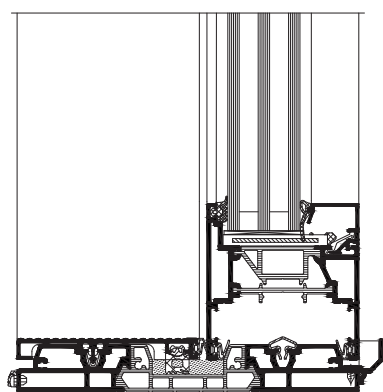
Soglia ribassata 25 mm Versione a una, due e tre rotaie Ideale per la ristrutturazione
