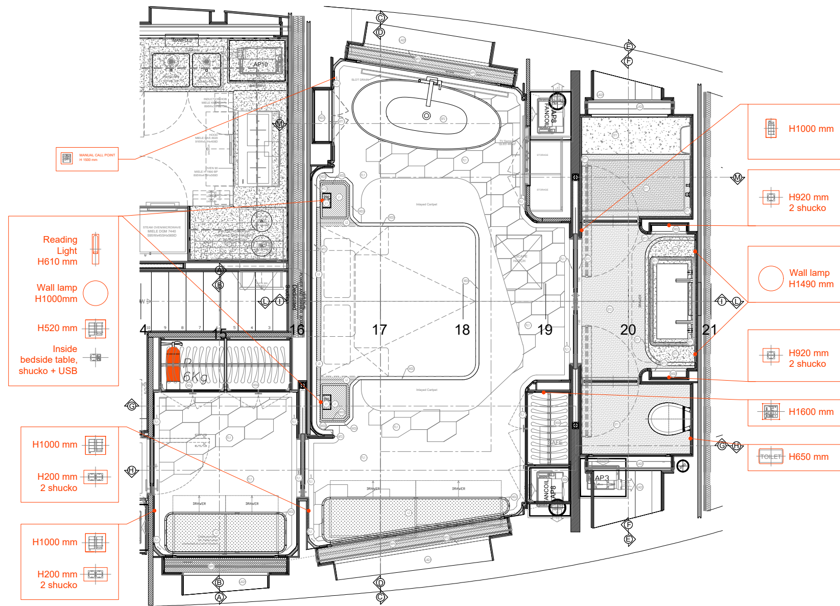
3 ELECTRICAL PLAN Scale: 1:20
