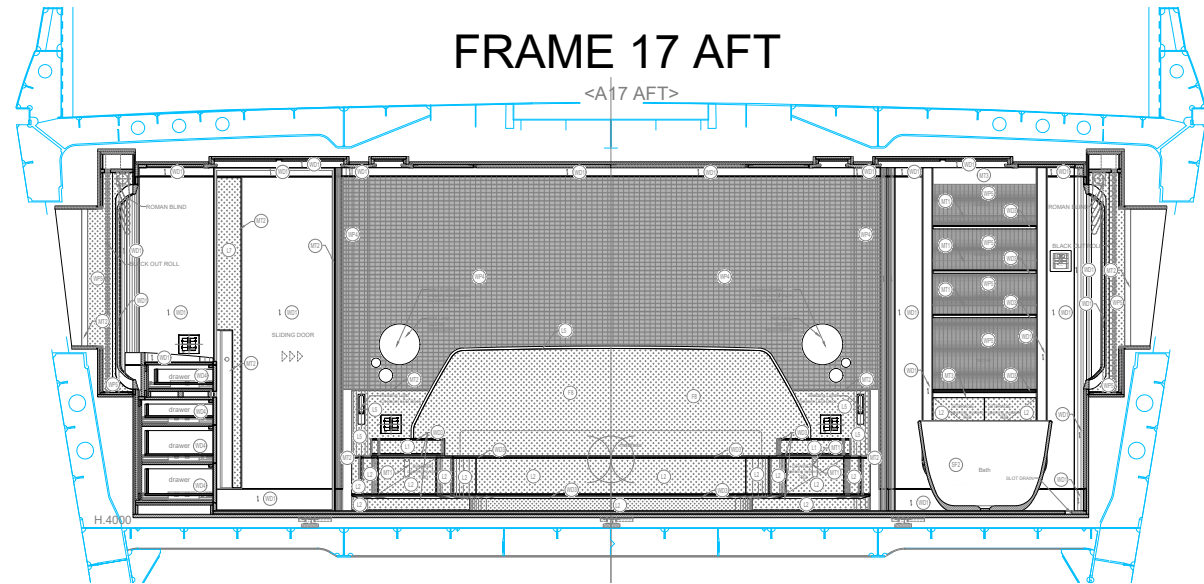
7 SECTION D Scale: 1:20
