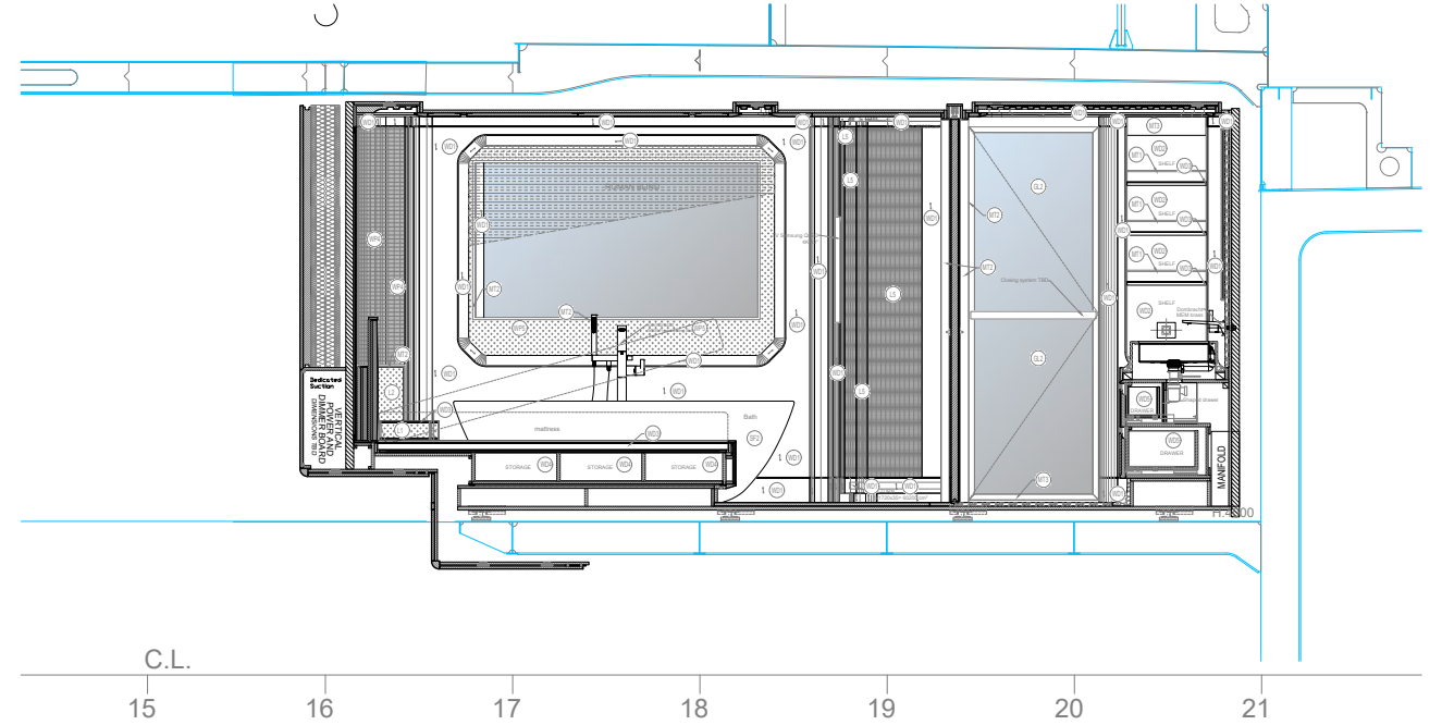
12 SECTION I Scale: 1:20
