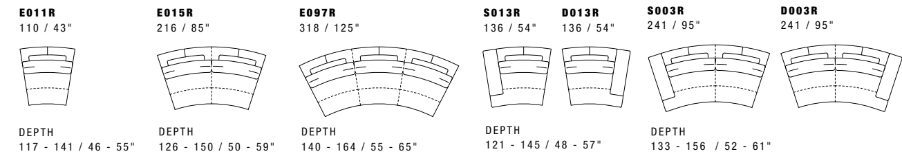
GROUP J Tutti gli elementi del Gruppo J hanno lo stesso modulo di seduta. All items in Group J have the same seat width
